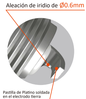
Bujía de iridio y Platino
